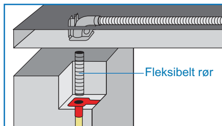
Forbindelse mellem præfabrikerede vægge og pladelofter
