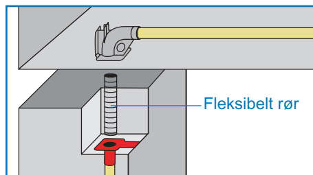
Forbindelser mellem præfabrikerede vægge og massive lofter.
