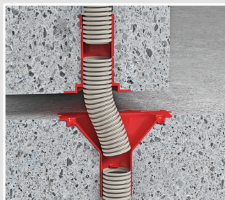
Udligning i længderetning \pm 20 mm.
