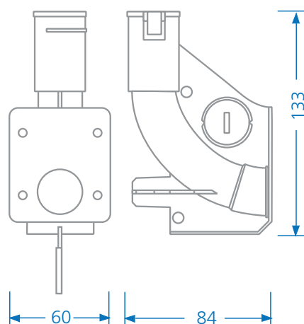
Væg-loft-overgang 90°
