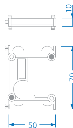
Udvidelseselement/ base
